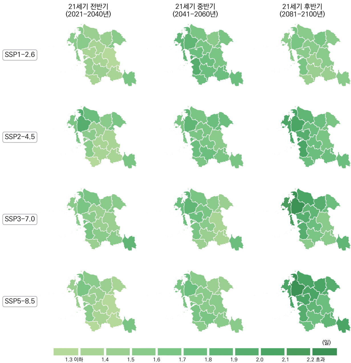
그림 4-39. 충청남도의 99퍼센타일강수일수(일) 전망 분포도
