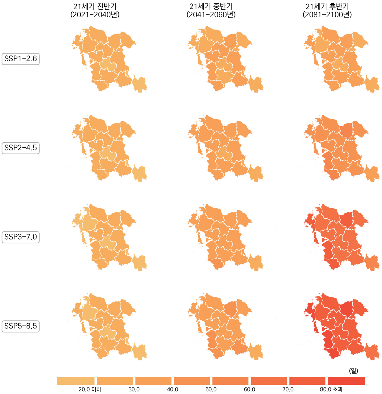
그림 4-19. 충청남도의 열대야일수(일) 전망 분포도
