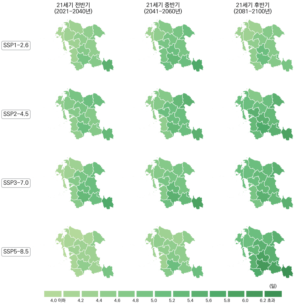
그림 4-38. 충청남도의 95퍼센타일강수일수(일) 전망 분포도
