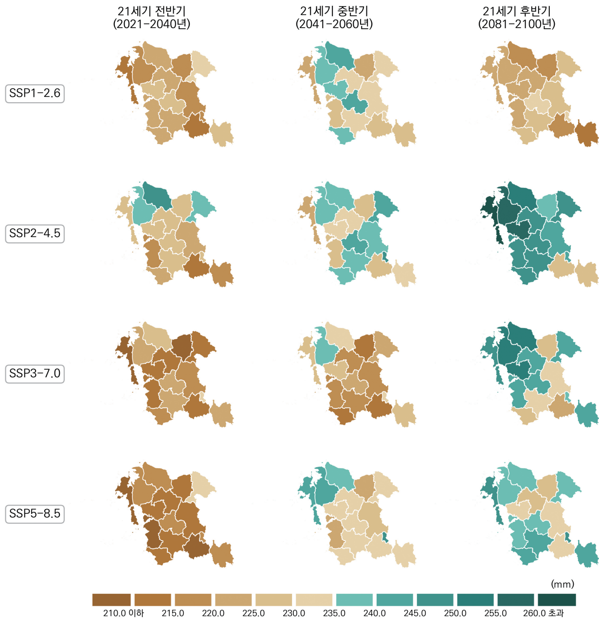
그림 4-37. 충청남도의 5일최다강수량(mm) 전망 분포도
