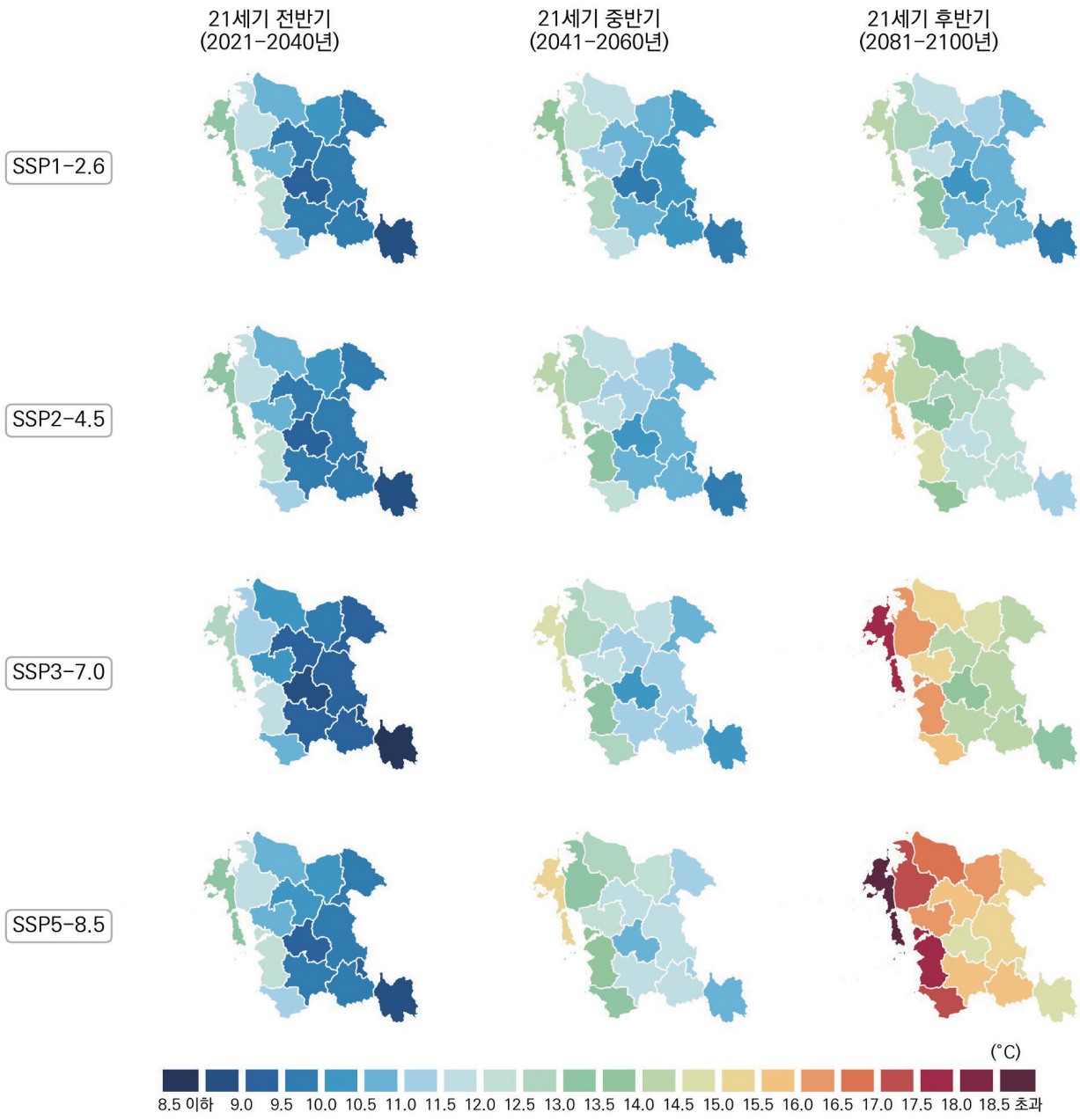
그림 4-14. 충청남도의 가을철 연평균 최저기온(°C) 전망 분포도
