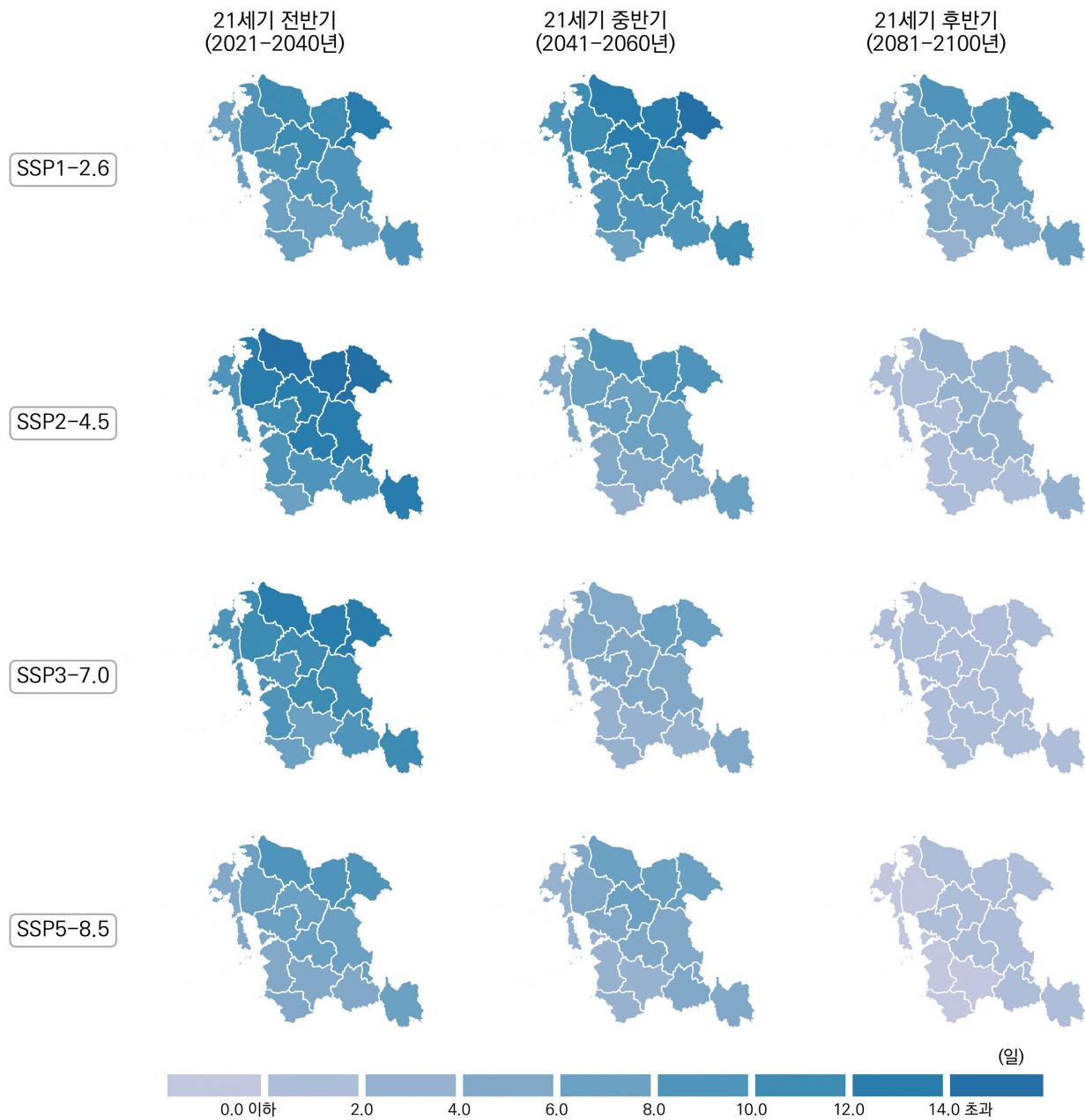
그림 4-28. 충청남도의 결빙일수(일) 전망 분포도
