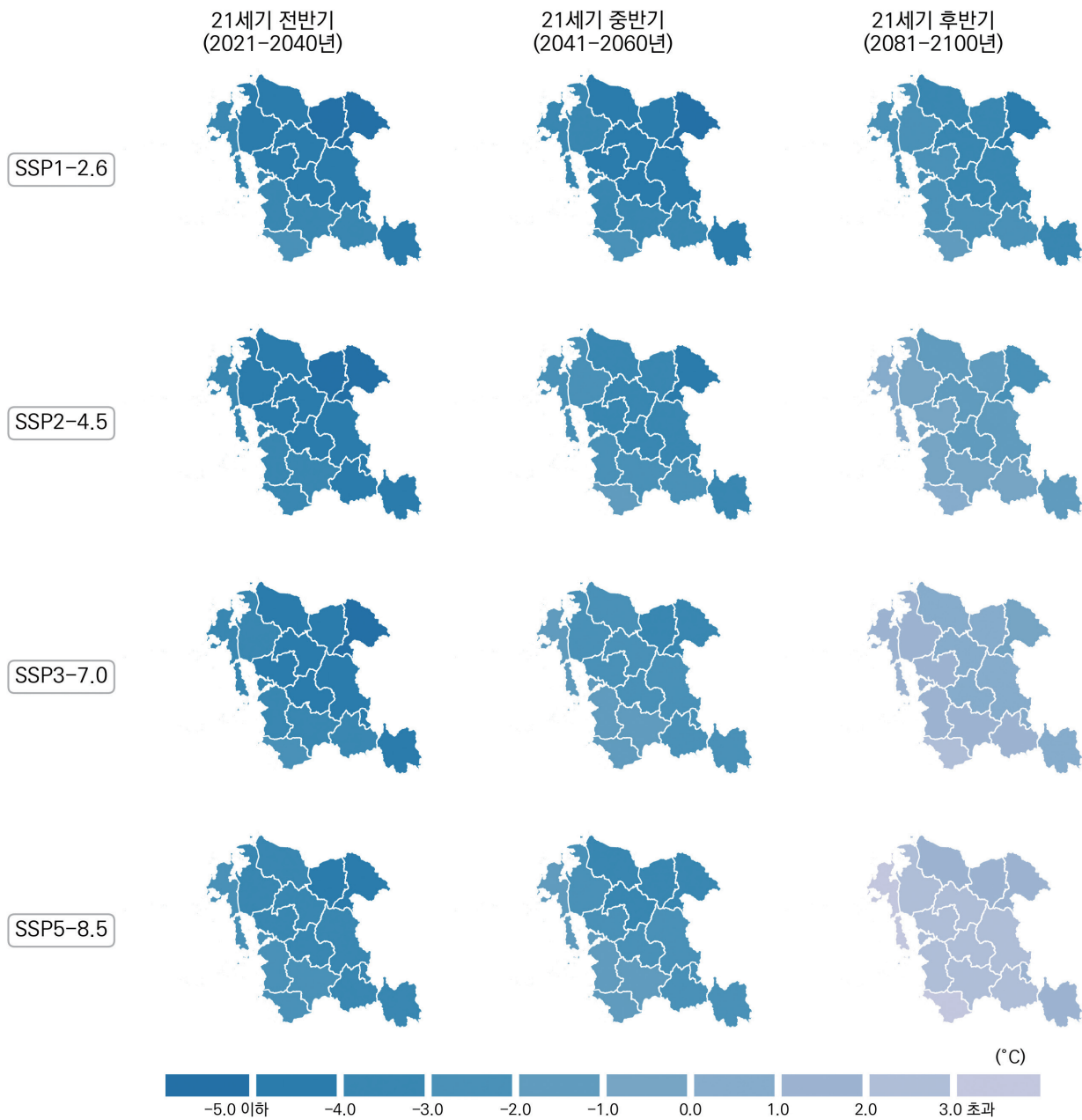
그림 4-32. 충청남도의 일최고기온 연최소(°C) 전망 분포도
