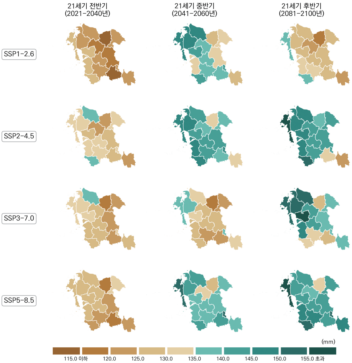
그림 4-36. 충청남도의 1일최다강수량(mm) 전망 분포도
