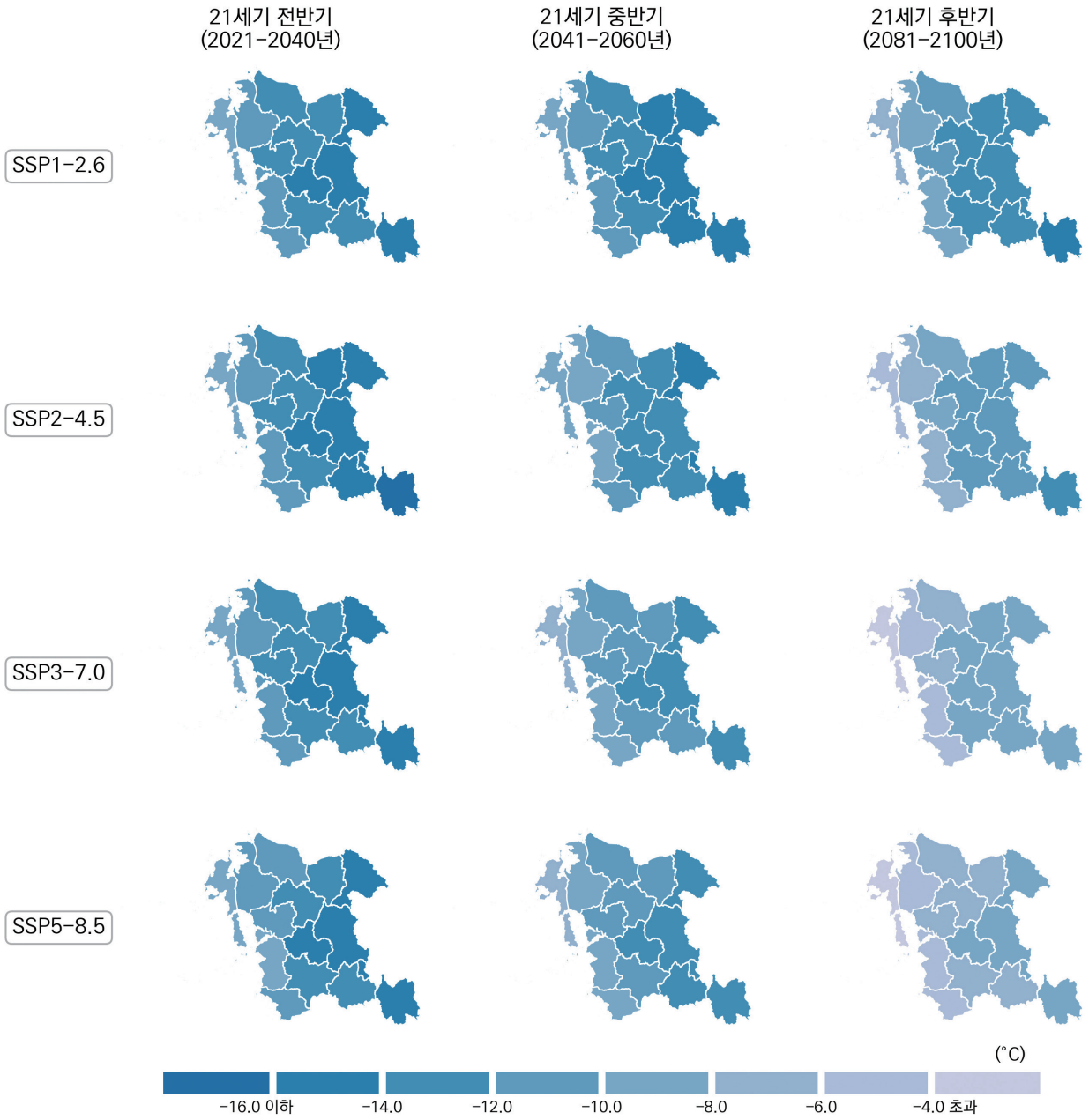
그림 4-33. 충청남도의 일최저기온 연최소(°C) 전망 분포도
