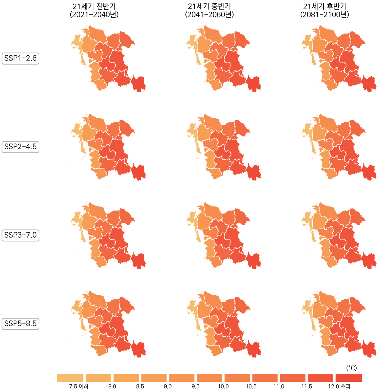
그림 4-25. 충청남도의 일교차(°C) 전망 분포도
