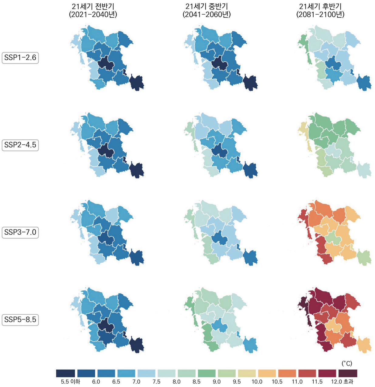
그림 4-12. 충청남도의 봄철 연평균 최저기온(°C) 전망 분포도
